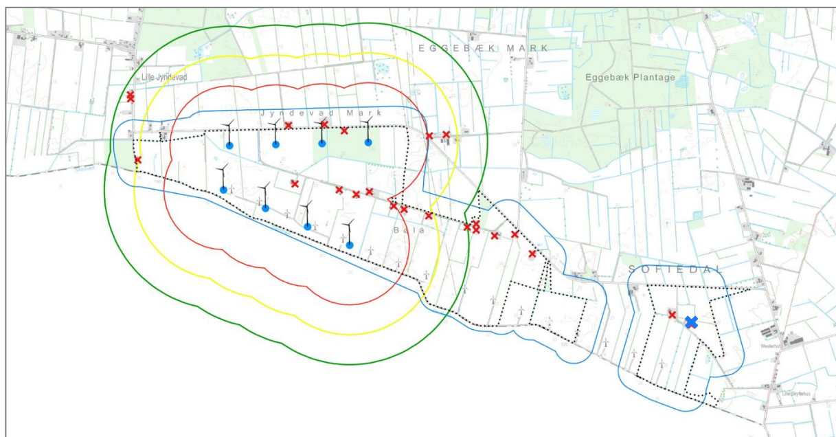
Figur 5 Afstande fra vindmøller til boliger. Boliger, markeret med rødt kryds, forventes nedlagt. Hvis Grænsevejen 13 (markeret blåt kryds) opretholdes, vil der blive etableret en passende afstand til boligen.
