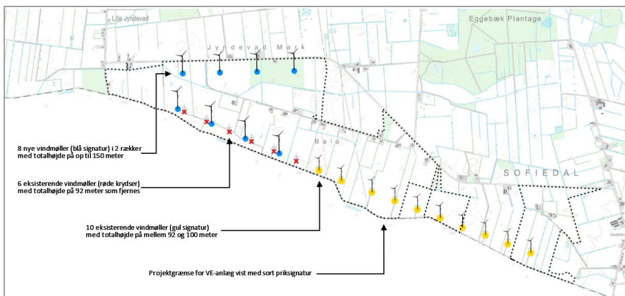
Figur 4 Nye og eksisterende vindmøller.
