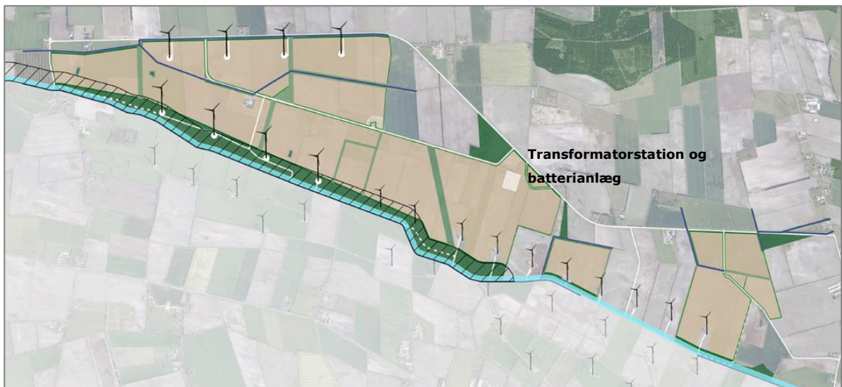
Figur 7 Placering af transformatorstation og batterianlæg markeret med lys brun signatur.
