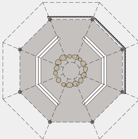
1:150 - Bålhytte
