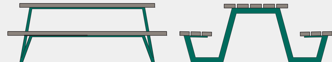
1:25 - Bordbænkesæt
