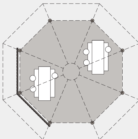
1:150 - Madpakkehus
