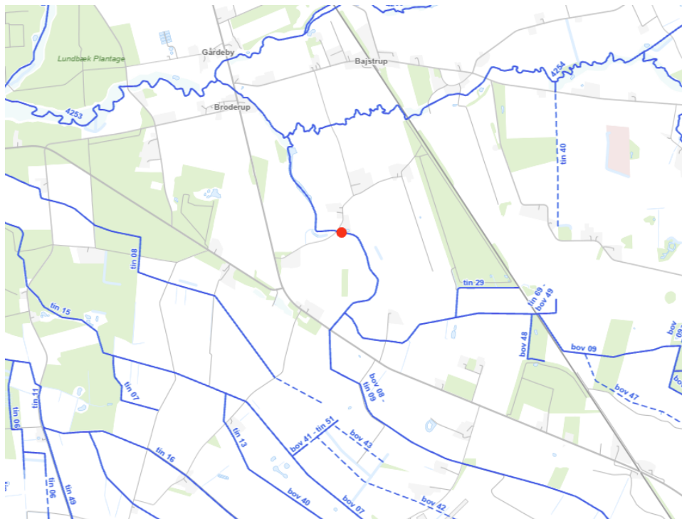
Figur 1: Rød markering opstrøms Gammel Bajstrupvej viser placering af sandfang. Sandfanget graves ud mod nord.
