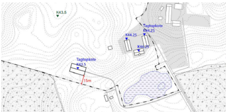
Situationsplan med terrænkoter
