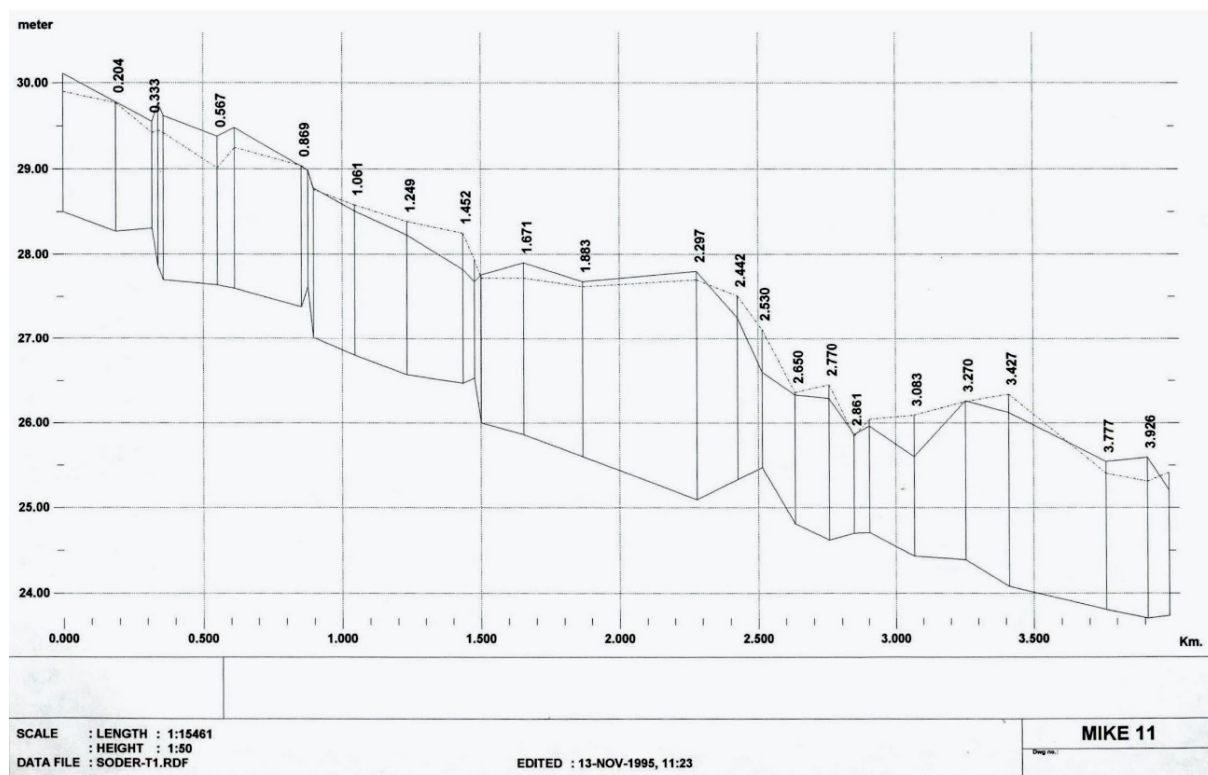
Figur 2: Den opmåling af vandløbet som er lagt til grund for projektet med etablering af okkersøen. Figuren er desuden vedlagt i større format som bilag til denne afgørelse.
