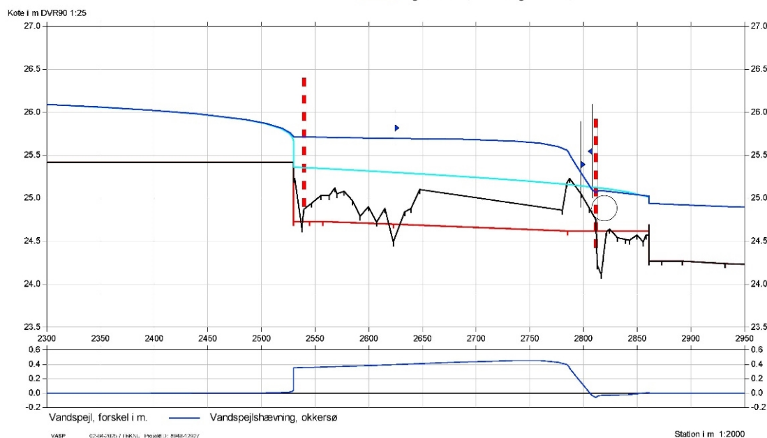
Figur 4: Figuren viser samme vandspejlsberegning som figur 3, men fokuseret omkring okkersøen. Under længdeprofilet for vandspejlsberegningen er indsat et differenceplot der viser hvor meget vandspejlet er hævet som følge af etablering af okkersøen. Figuren er desuden vedlagt i større format som bilag til denne afgørelse.
