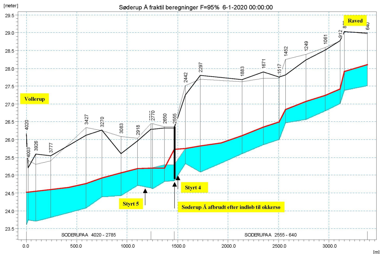
Figur 1: Figuren fra afgørelsen af 2019 som klagenævnet baserer hjemvisning af sagen på. Hverken stationering eller de forskellige labels, pile og beskrivelser er indtegnet korrekt på figuren. Figuren er desuden vedlagt i større format som bilag til denne afgørelse.
