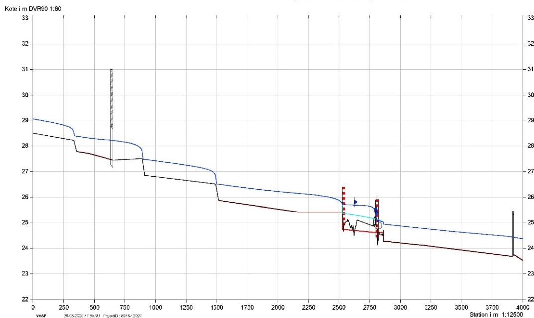
Figur 3: Figuren viser en vandspejlsberegning ved en vandføring på 504 l/s, som anvendt i afgørelsen af 2019, for Søderup Å med hhv. regulativmæssig skikkelse inden etablering af okkersøen og regulativmæssig skikkelse med indlagt okkersø, som opmålt i februar 2025. Figuren er desuden vedlagt i større format som bilag til denne afgørelse.
