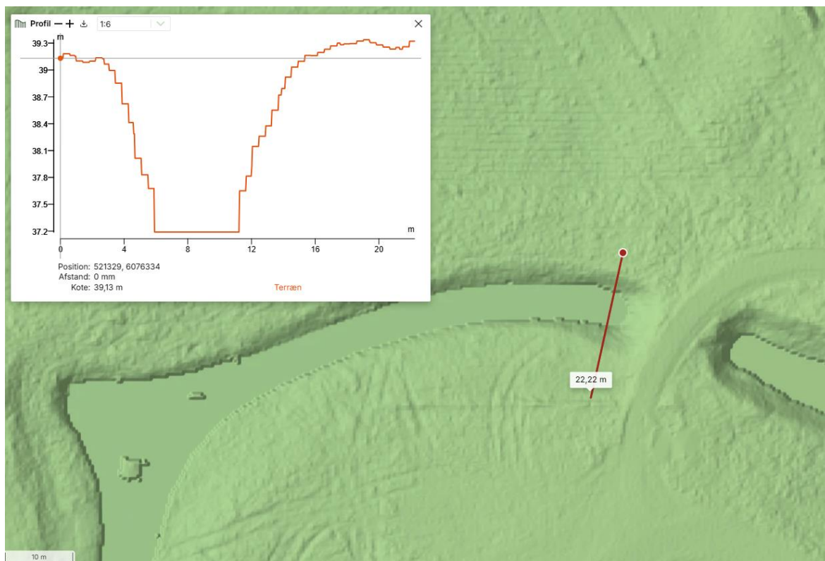
Figur 1: Højdemodel over vandløbet i området.
