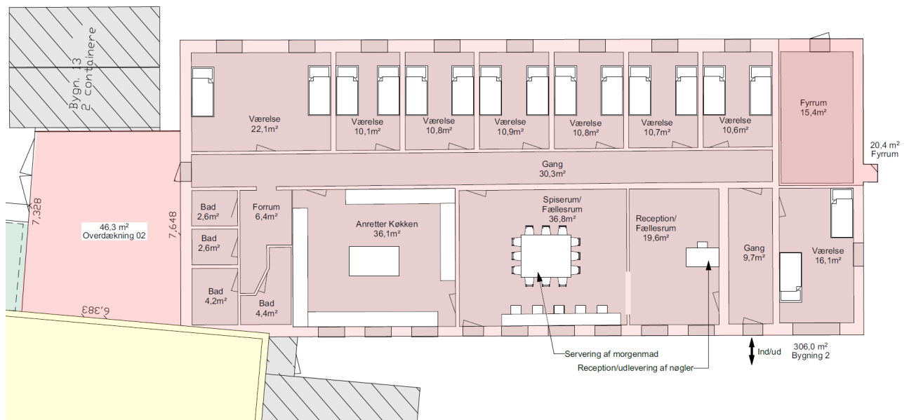
Plantegning med spiseområde og reception
